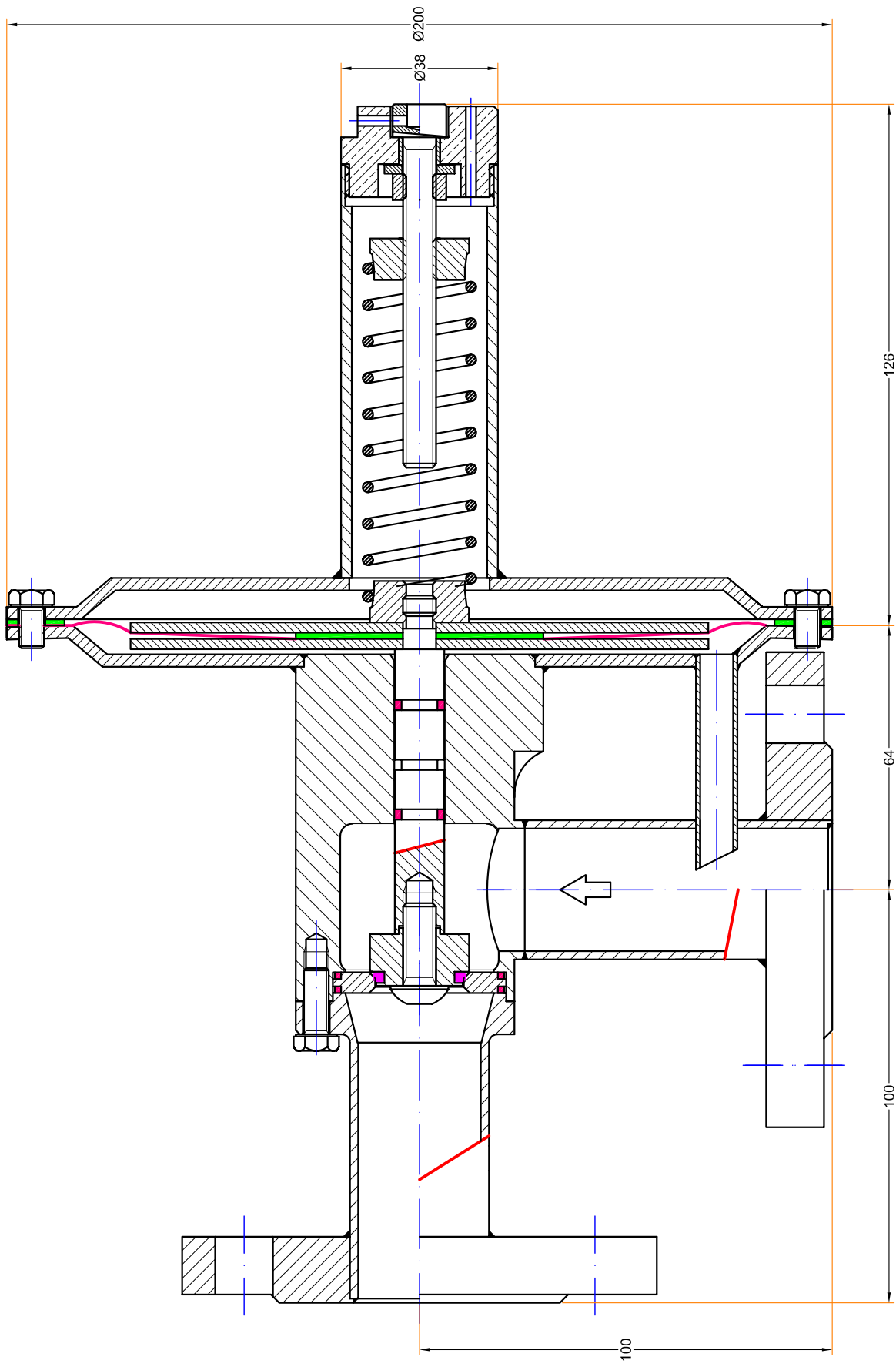
DÉVERSEUR en équerre Edge RELIEF VALVE
